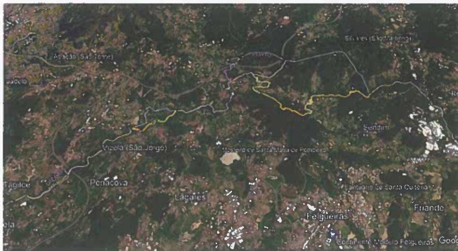
Figura 1 – Extensão e localização da requalificação dos Rios Vizela, Bugio e Ferro
