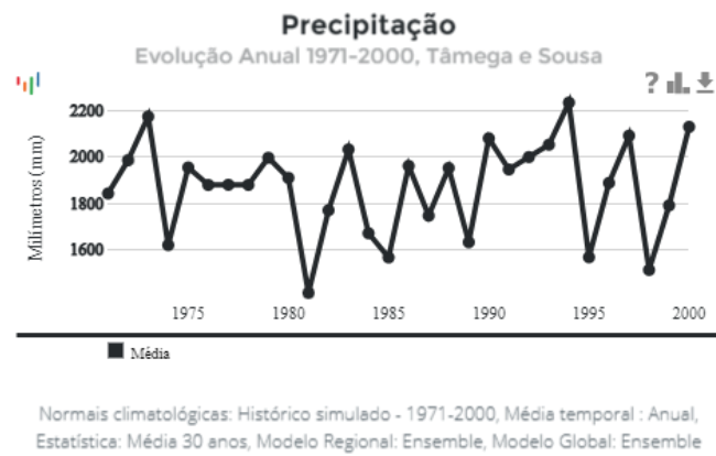
Figura 28. Evolução da precipitação média acumulada na sub-região do Tâmega e Sousa, para o período 1971-2000 Fonte: Portal do Clima
